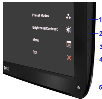
Bedienelemente an der Vorderseite
